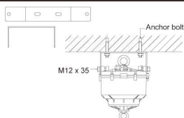
混凝土顶棚安装
