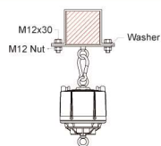
四角管道安装
