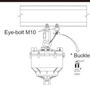
C型钢安装
